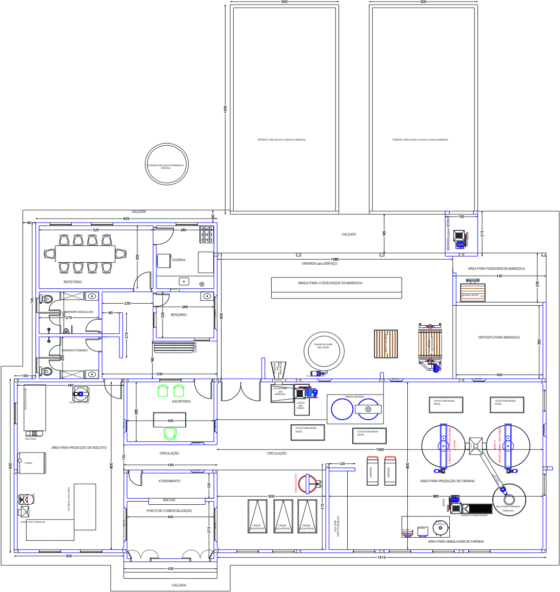
PLANTA BAIXA E LEY-OUT DE EQUIPAMENTOS
